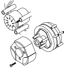
Filterüberwachung, Druckdifferenzschalter
